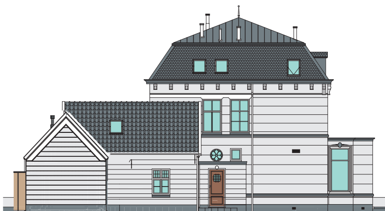
Linker zijgevel
